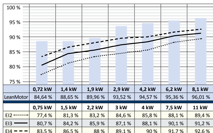
Rendement du LeanMotor par rapport aux moteurs asynchrones
