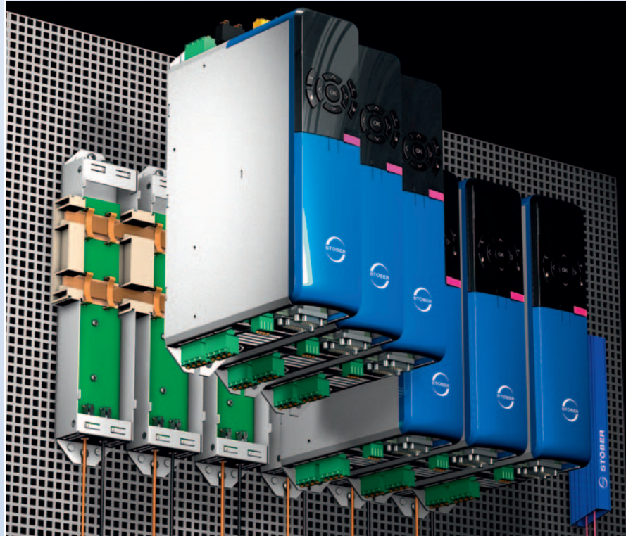
SD6 mit Quick DC-Link zur Zwischenkreiskopplung, ergänzt durch einen Bremswiderstand.
